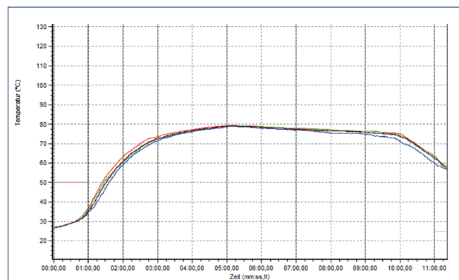
Temperaturkurve
